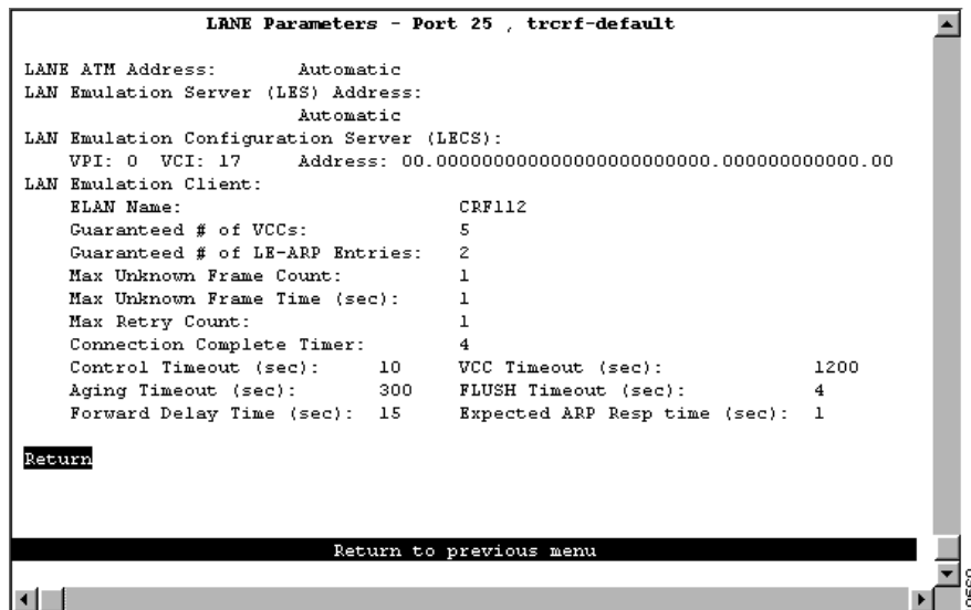
Figure 10-4 LAN Parameters Panel
